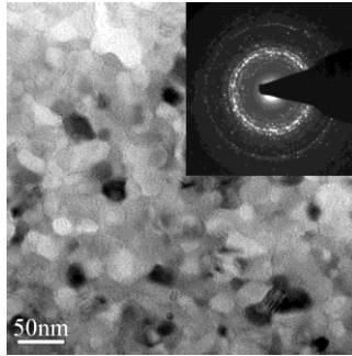
图 1-1 热处理后的磁体的 TEM 照片及 SAED 图像
